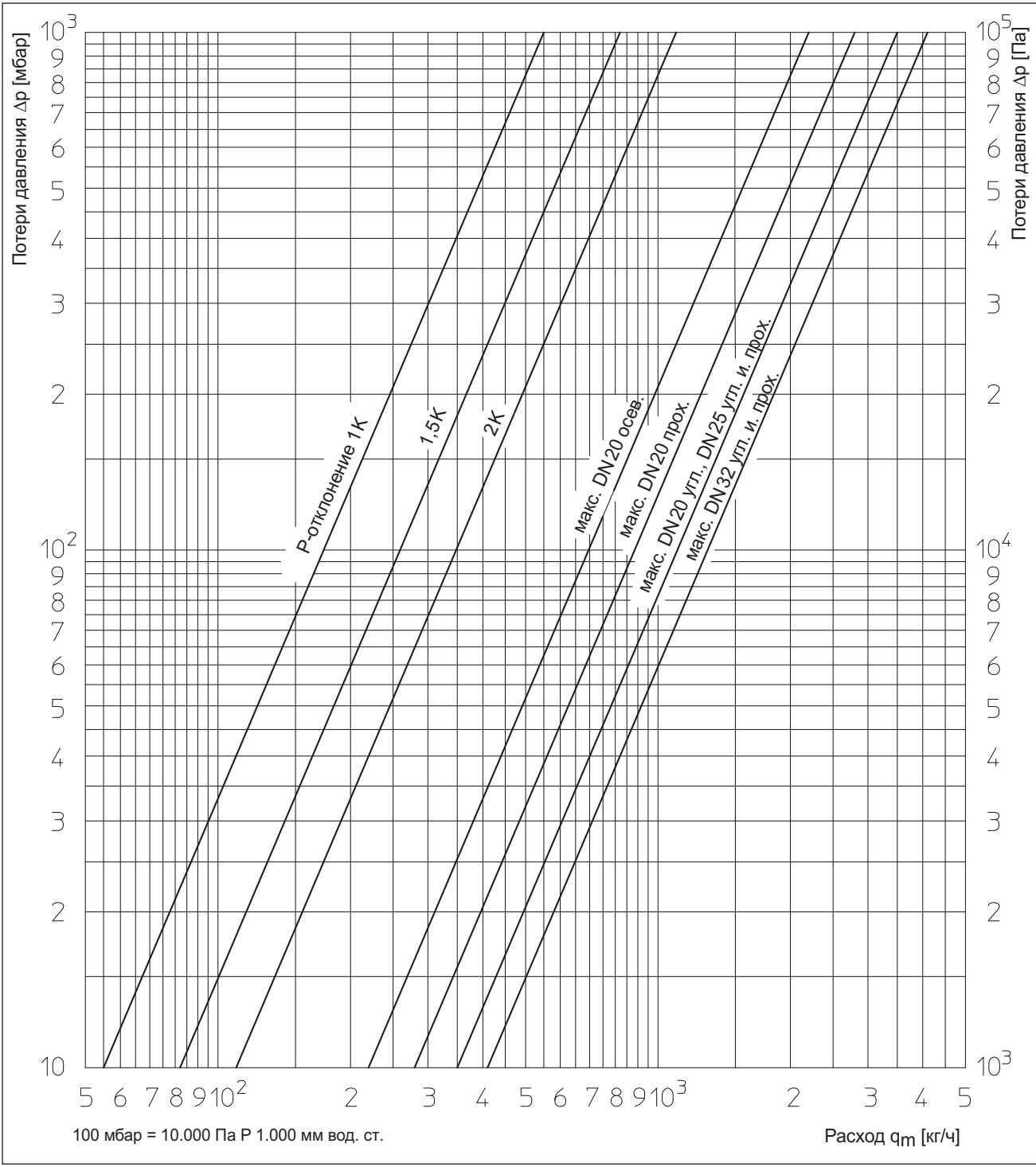
Диаграмма 3 Термостатические вентили Oventrop серий „А“ и „RF“, DN 20-DN 32 Все исполнения, Р-отклонение от 1 до 2 К и Kvs
