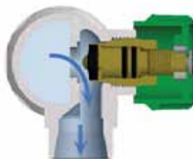
Рис. 18. MultiFAR Регулирующий коллектор
