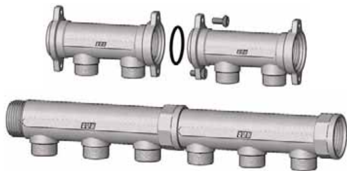
Рис. 3. Соединения коллекторов
