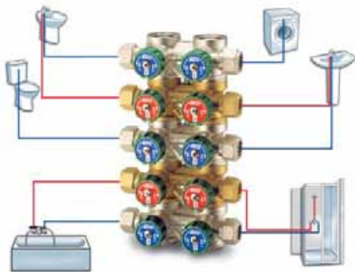
Рис. 5. Подключение регулируемого параллельного коллектора
