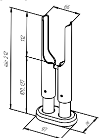
рис. 1 Регулируемый напольный кронштейн 2-х колончатый
