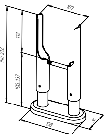
рис. 2 Регулируемый напольный кронштейн 3-х колончатый
