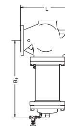
VFG 2 DN 150 - 250 t_{max} 200\text{ }^{\circ}\text{C}
